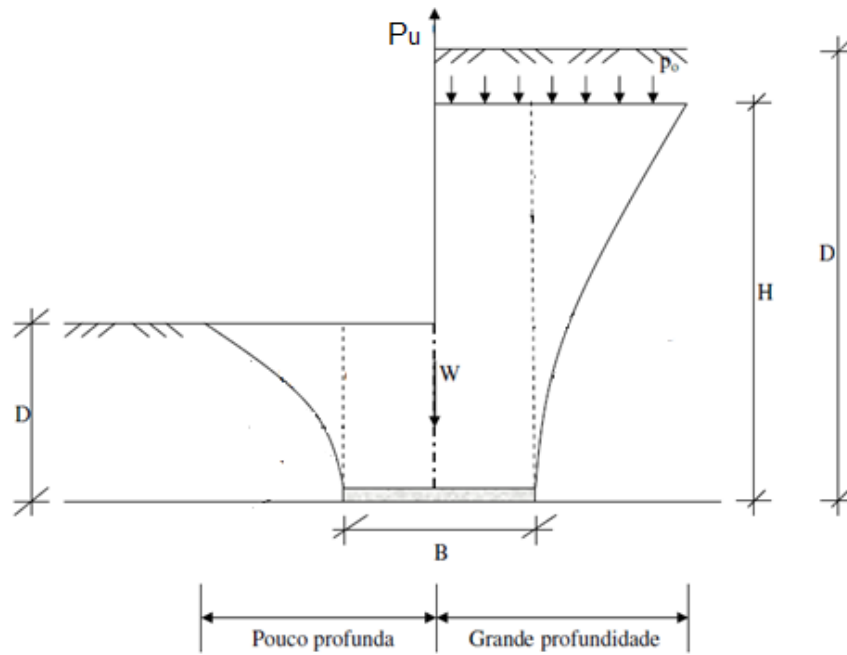
Figura 2.15 – Superfície de ruptura acima da ancoragem
