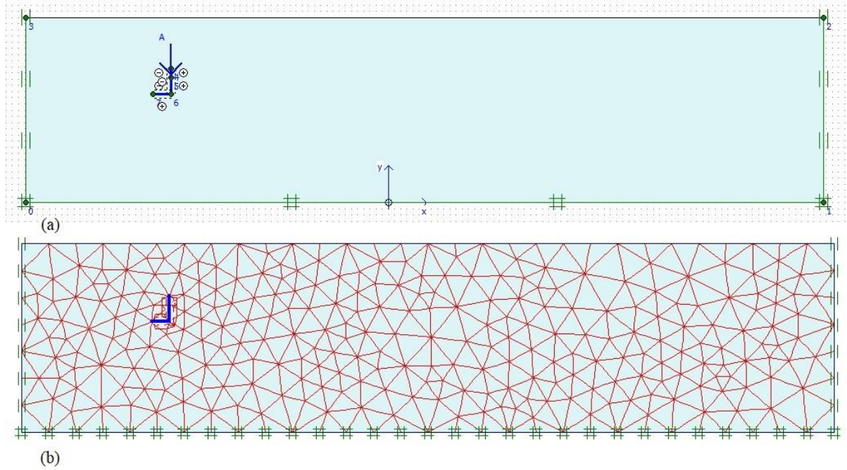
Figura 3.25 – Interfaces do PLAXIS 2D (a) modelo geométrico de estado plano de tensão para D/h = 3 e (b) malha fina de elementos finitos associada
