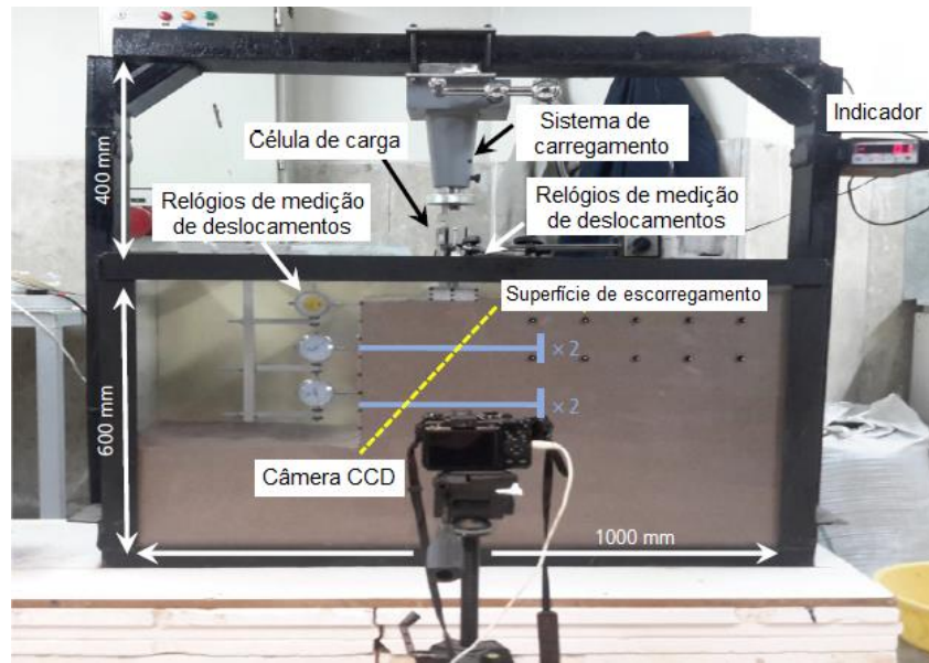
Figura 2.42 – Tanque experimental e câmera CCD
