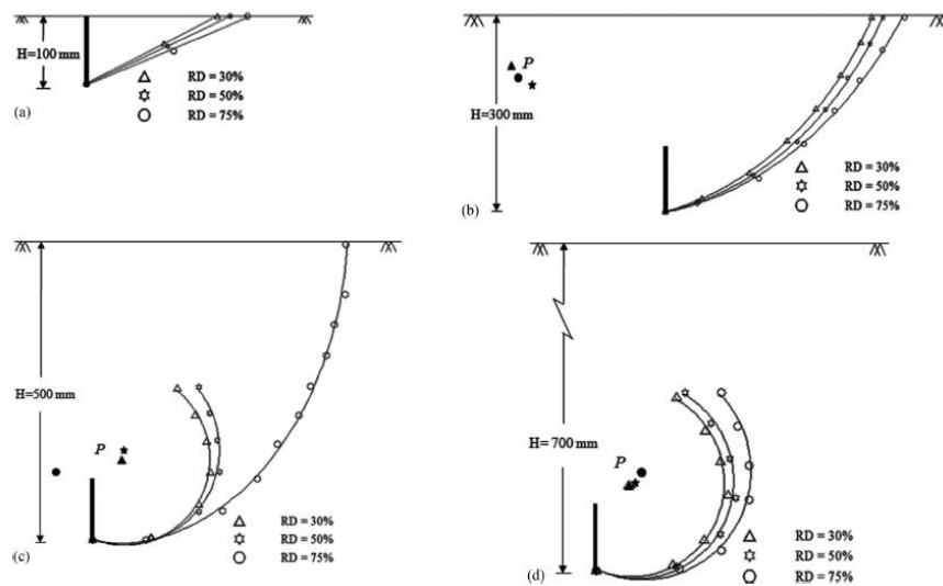
Figura 2.10 – Delineado das superfícies de ruptura: (a) H/h = 1 ; (b) H/h=3 ; (c) H/h=5 e (d) H/h=7
