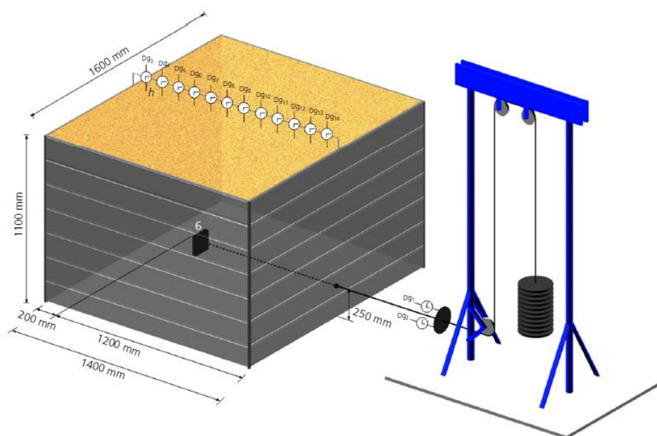
Figura 2.24 – Esquema de ensaio em modelo reduzido 1g
