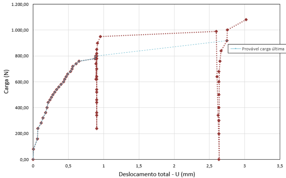
Figura 4.7 – Curva carga x deslocamento para ancoragem 03, D/h=3, sobrecarga q_3 = 4,415 \text{ kPa}
