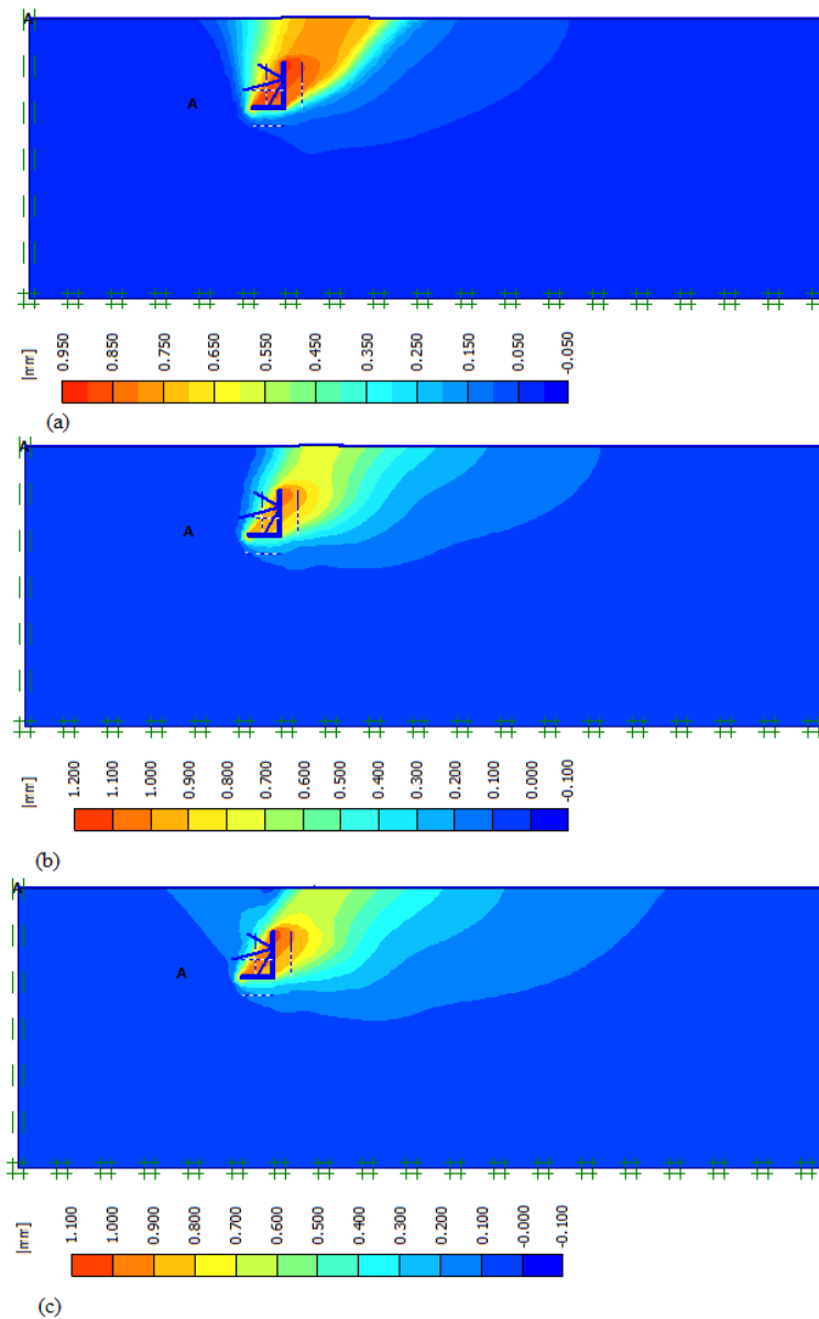
Figura 4.42 – Modificação dos deslocamentos totais com o aumento da sobrecarga (a) q = 0,000 kPa, (b) q = 2,077 kPa e (c) q = 3,890 kPa
