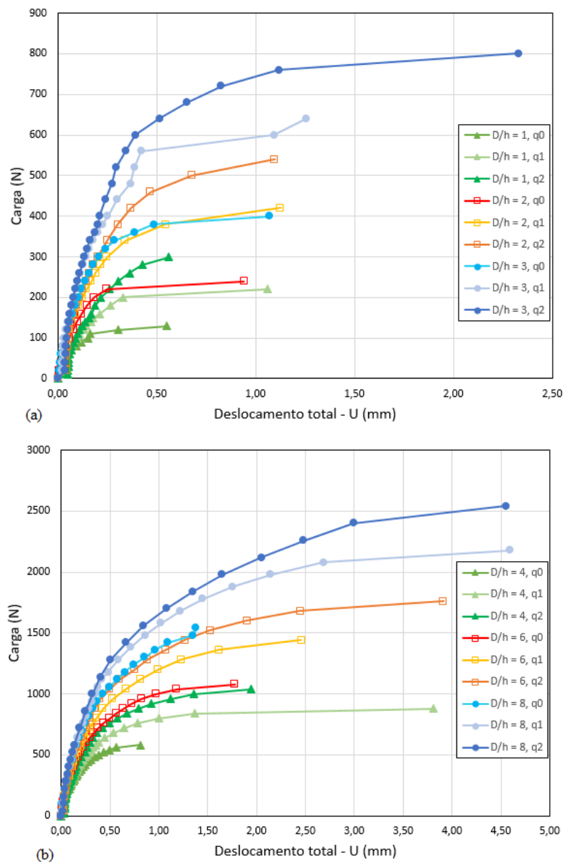
Figura 4.41 – Influência da sobrecarga nos deslocamentos para ancoragem 01, \theta = 15^\circ nas profundidades (a) D/h = 1, 2 e 3 e (b) D/h = 4, 6 e 8
