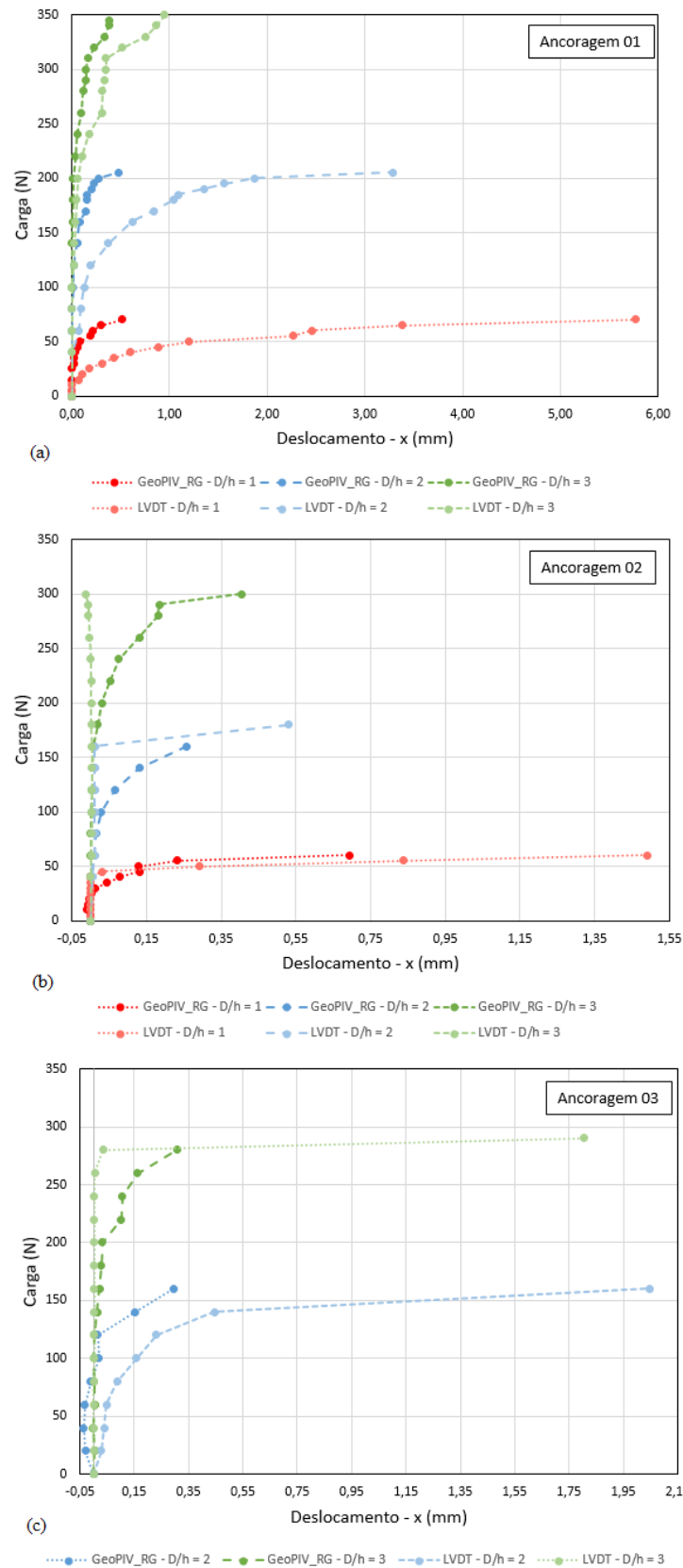
Figura 4.2 – Deslocamentos horizontais medidos pelo LVDT e GeoPIV-RG referentes à (a) ancoragem 01, (b) ancoragem 02 e (c) ancoragem 03
