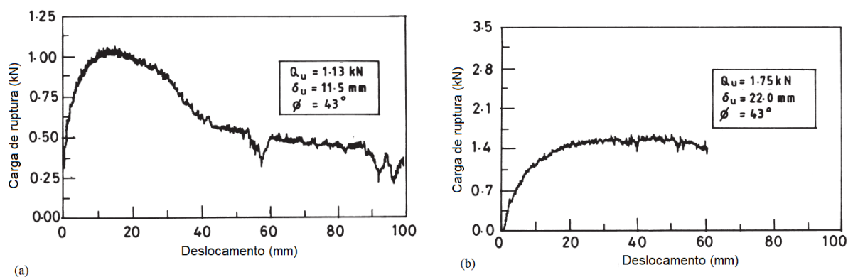
Figura 2.30 – Curva carga x deslocamento para (a) D/B = 3,9 , ruptura generalizada e (b) D/B = 6,99 , ruptura localizada
