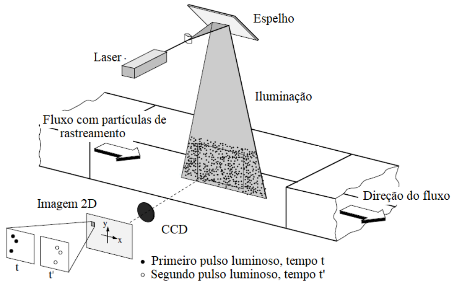
Figura 2.31 – Arranjo experimental para PIV em túnel de vento
