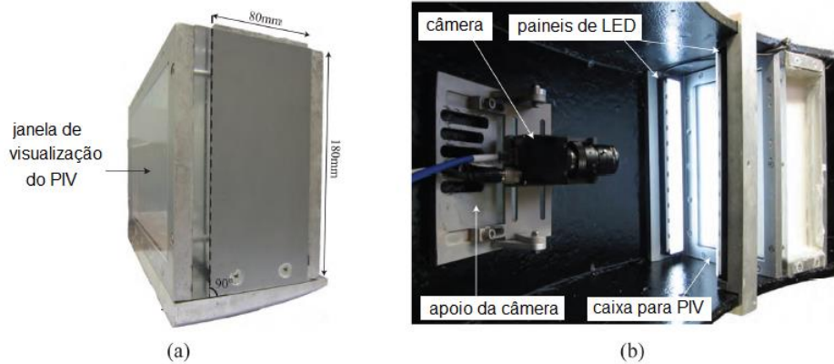
Figura 2.38 – Esquema para realização de ensaio em centrífuga e aplicação da técnica PIV (a) caixa do ensaio e (b) esquema de luz e câmera
