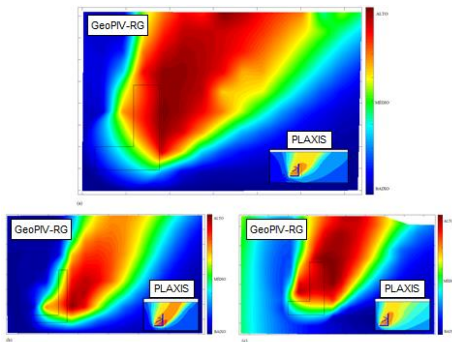
Figura 4.23 – Campo de deslocamentos total para D/h = 2 (a) ancoragem 01, (b) ancoragem 02 e (c) ancoragem 03
