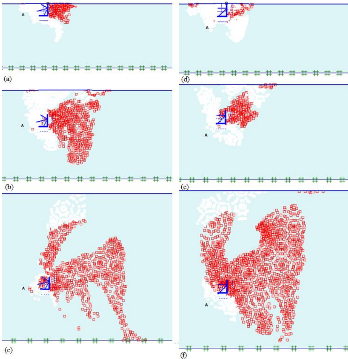
Figura 4.32 – Pontos de plastificação e ruptura a tração para ancoragem 01, \theta = 15^\circ (a) D/h = 1 , (b) D/h = 3 e (c) D/h = 8 e \theta = 45^\circ (d) D/h = 1 , (e) D/h = 3 e (f) D/h = 8 e
