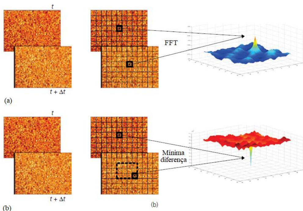
Figura 2.34 – Diagrama esquemático da análise PIV no (a) domínio da frequência e (b) domínio espacial
